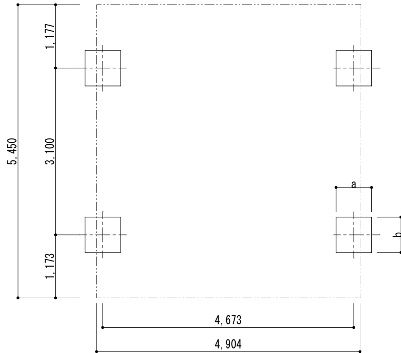
■ 基礎配置図
